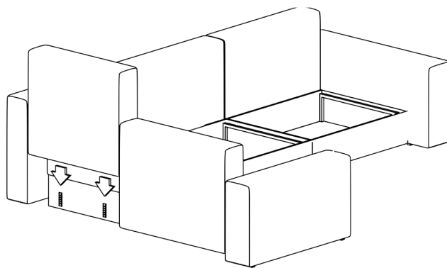
4. Прикрепить спинку соединителями папа/мама
